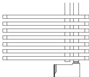
Desni priključak 50 mm
